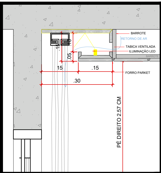
DET. 09 - CORTINEIRO ILUMINADO COM RETORNO DE AR 1:10
