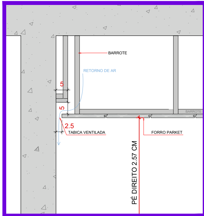
DET. 02 - TABICA SIMPLES COM RETORNO 1:10
