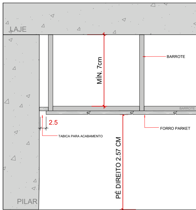
DET. 01 - TABICA SIMPLES 1:10
