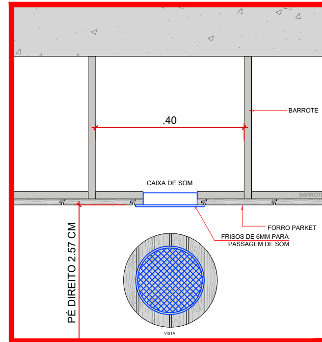
DET. 06 - CAIXA DE SOM 1:10
