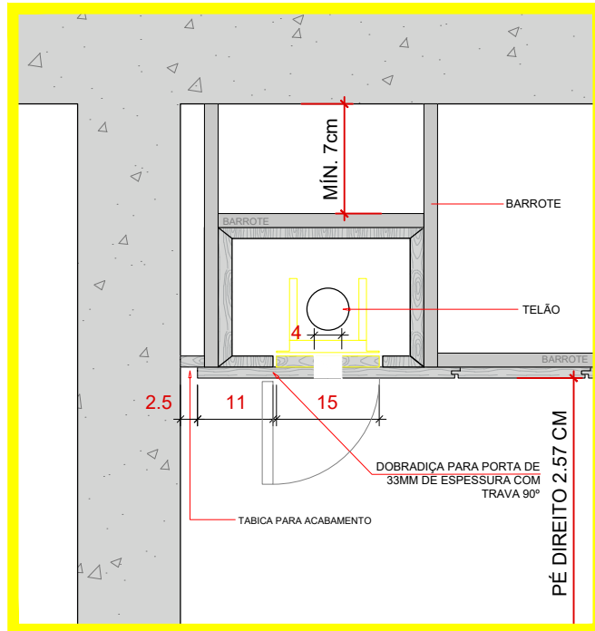
DET. 04 - TELÃO EMBUTIDO 1:10
