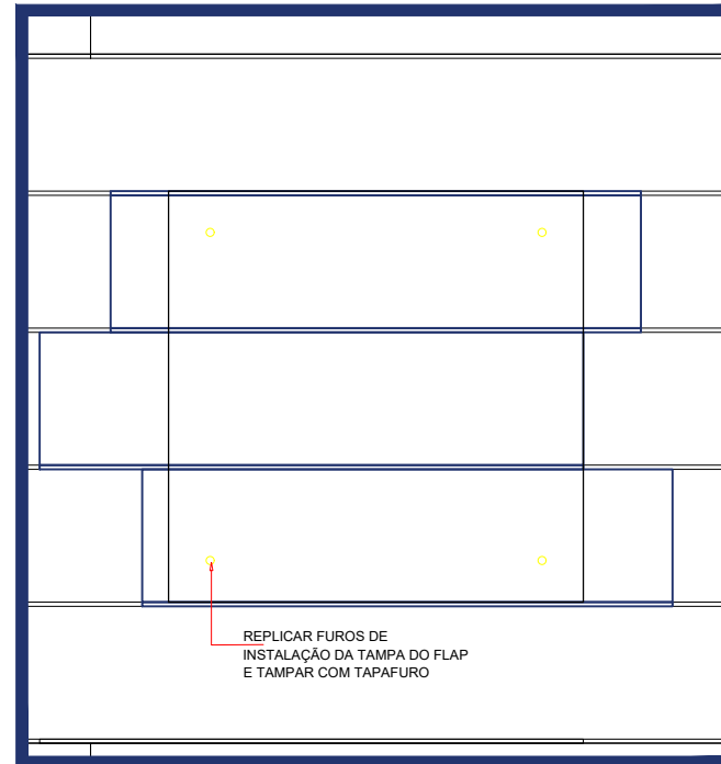
DET. 08 - FLAP PROJETOR 1:10
