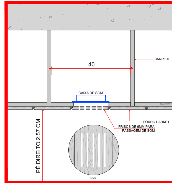
DET. 07 - CAIXA DE SOM 1:10
