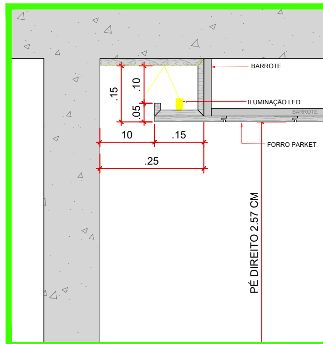
DET. 11 - SANCA ILUMINADA 1:10
