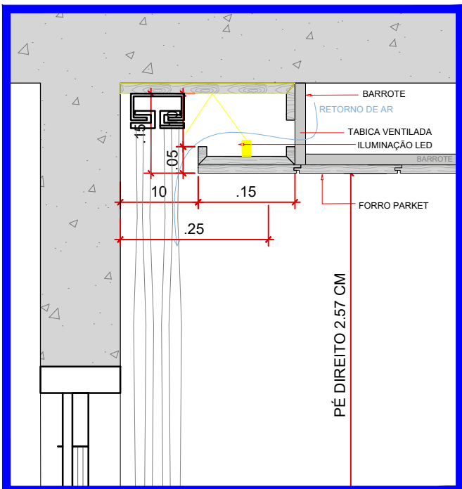
DET. 10 - CORTINEIRO ILUMINADO COM RETORNO DE AR 1:10
